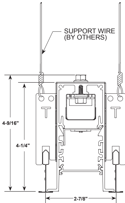
9/16 GRID
