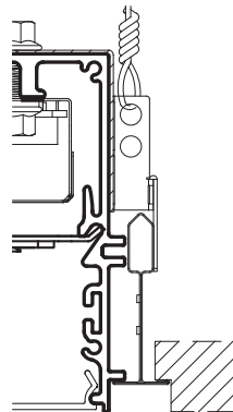
T9/16" GRID
