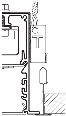
9/16" GRID
