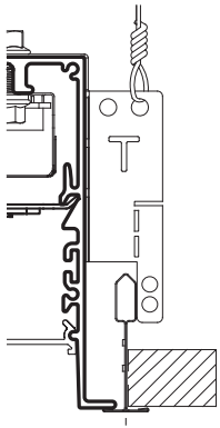
9/16" GRID
