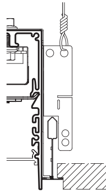
T9/16" GRID
