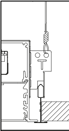
9/16 T-GRID
