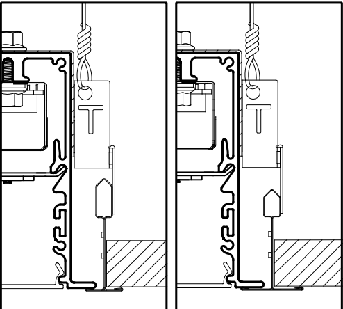
9/16 T-GRID
