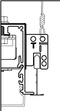
9/16 T-GRID
